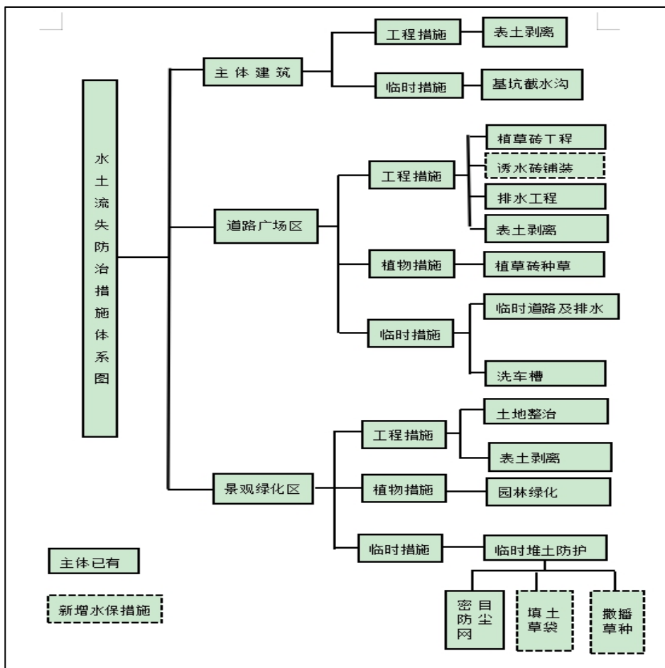
图3-1 水土流失防治措施体系图
