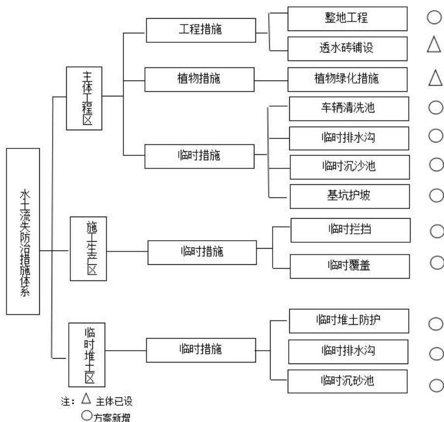
图 3-1 誉华金科瑞昌路141号专汽地块项目水土流失防治措施体系图
